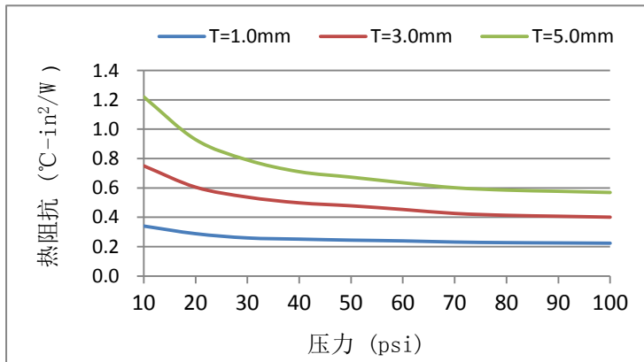
热阻抗
